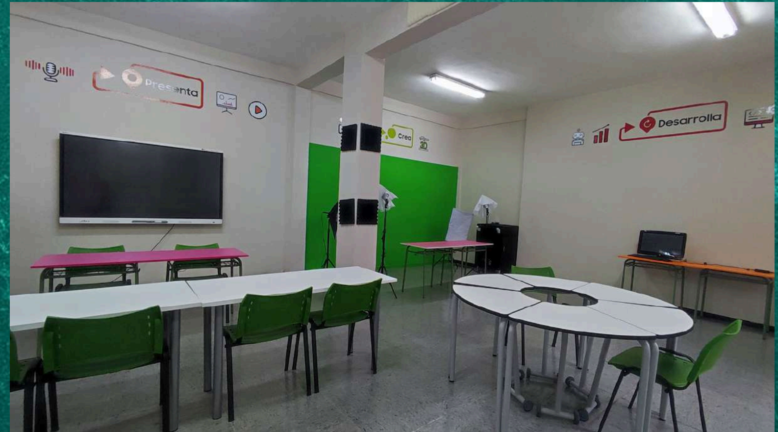
Espacio croma
